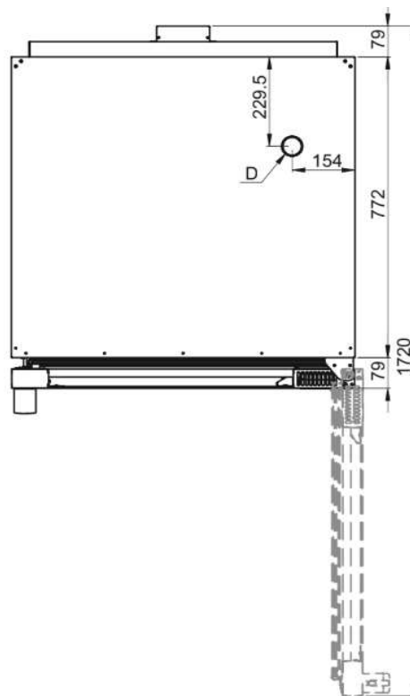
Vue de haut porte ouverte
